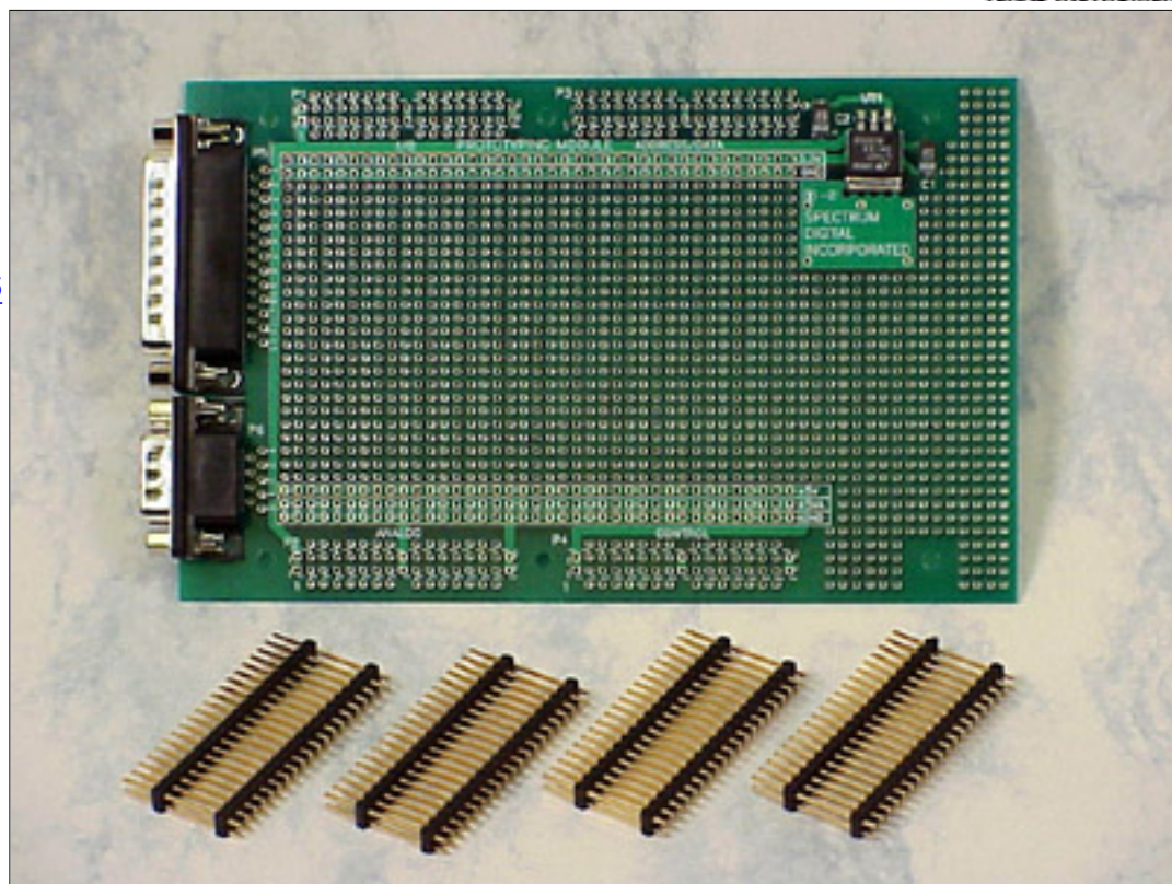
Prototyping Module
